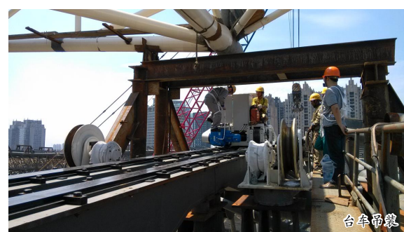
开合屋盖调试
